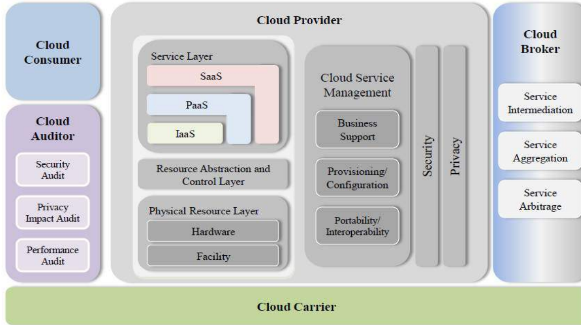
NIST-Cloud-Ref-Architecture
